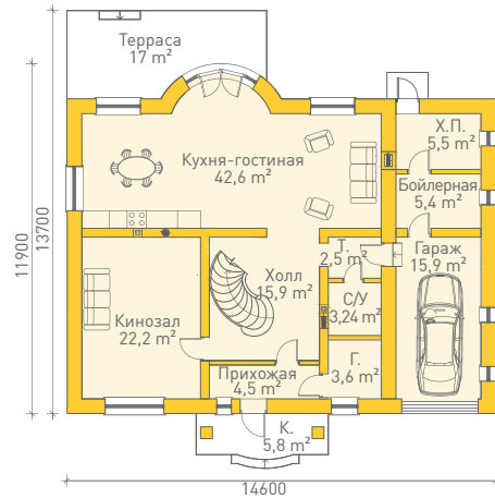
Экспликация | 1 этаж
