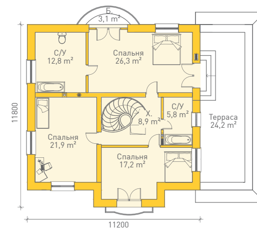
Экспликация | 2 этаж
