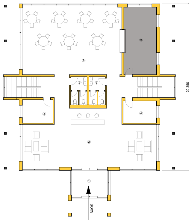
План | 1 этаж
